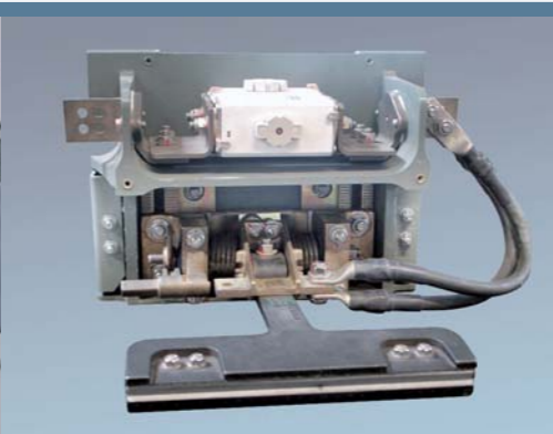
Dritte-Schiene Stromabnehmer, Kontaktierung von oben
