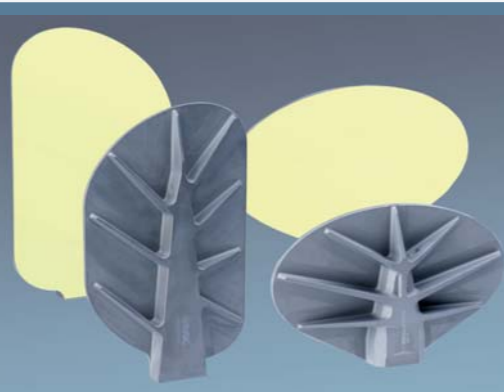
Hochleistungs-Scannerspiegel aus optoSiC ™ mit patentiertem Rippdesign
