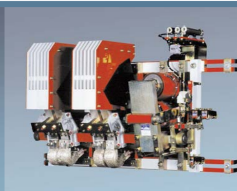
Gleichspannungs-Leistungsschütz
